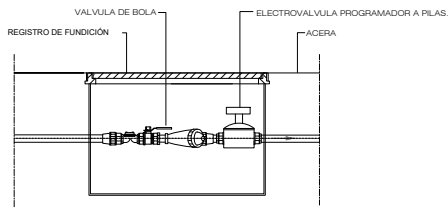
SECCION
