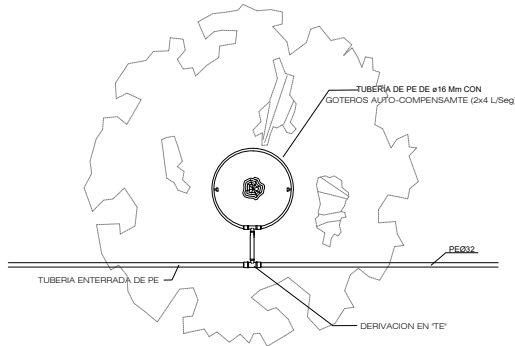
ALIMENTACIÓN ARBOL EN ZONAS VERDES
