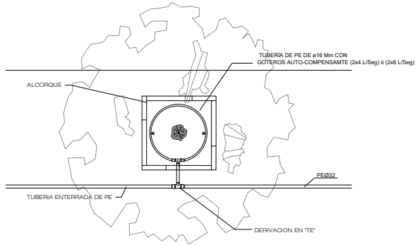
ALIMENTACION A ALCORQUE (S/E)
