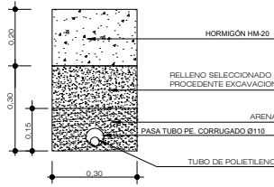
SECCION DE ZANJA PARA TUBERIA EN CRUCES BAJO CALZADAS
