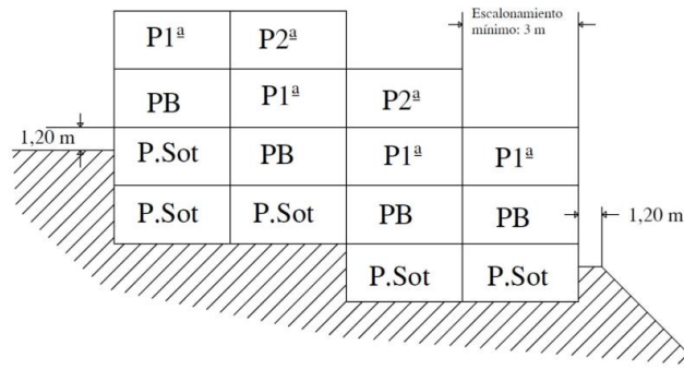
Esquema de sección de edificación
